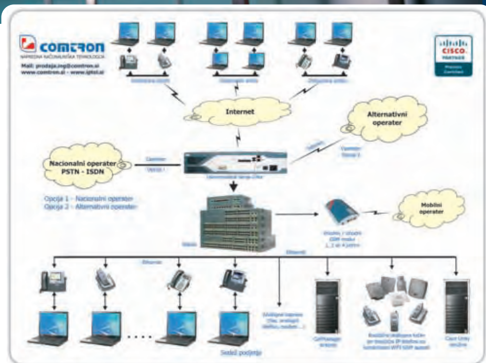
Postavitev UC Manager rešitev IP telefonije
